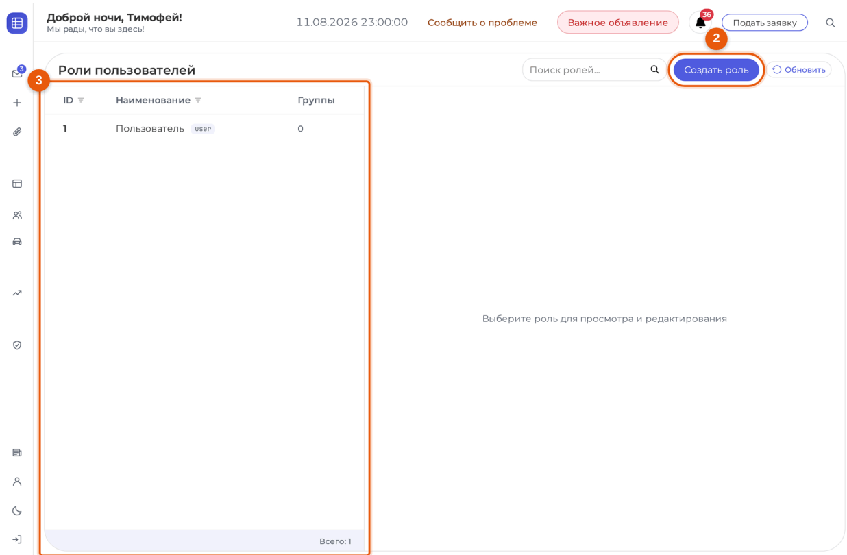
Рисунок 6.1 — Список ролей
